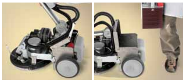
Vispa 35 B Il vano batteria è facile da raggiungere e permette una immediata sostituzione della batteria
